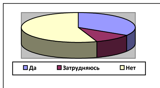
Рис. 1. Абстрактная идентификация
