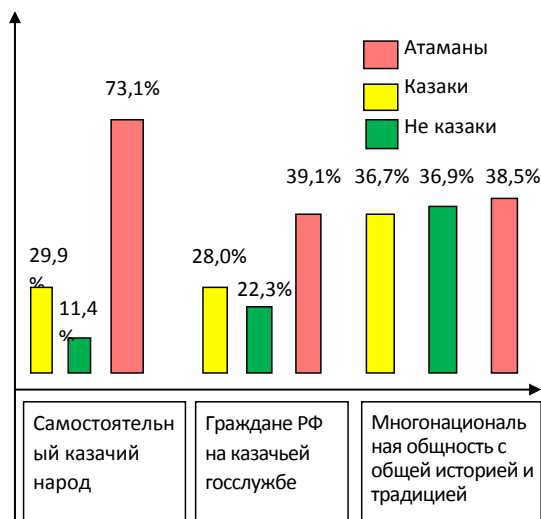
Рис. 2. Идентификационная категория
